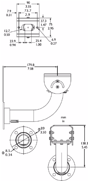
LTC 9215/00S Kurze Wandhalterung für den Inneneinsatz
