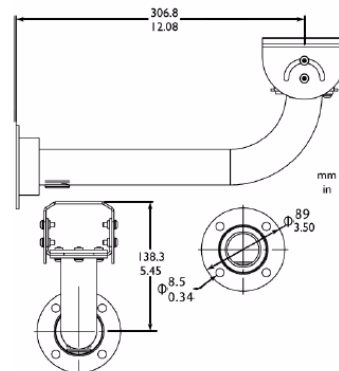
LTC 9215/00 Wandhalterung für den Außeneinsatz
