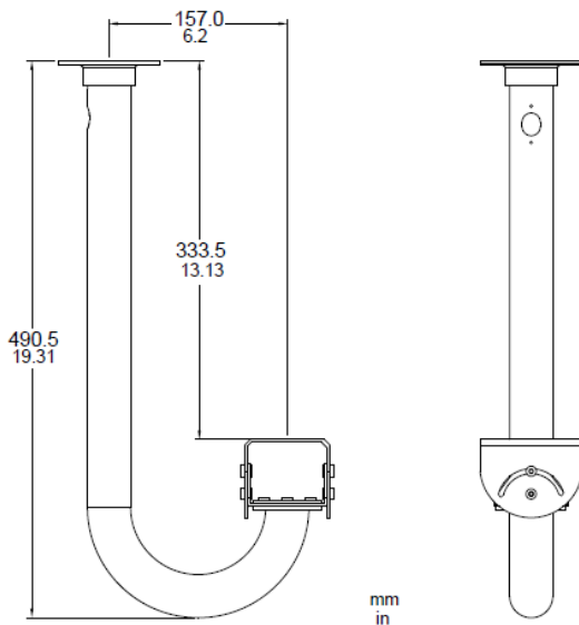
LTC 9215/00S Kurze Wandhalterung für den Inneneinsatz
